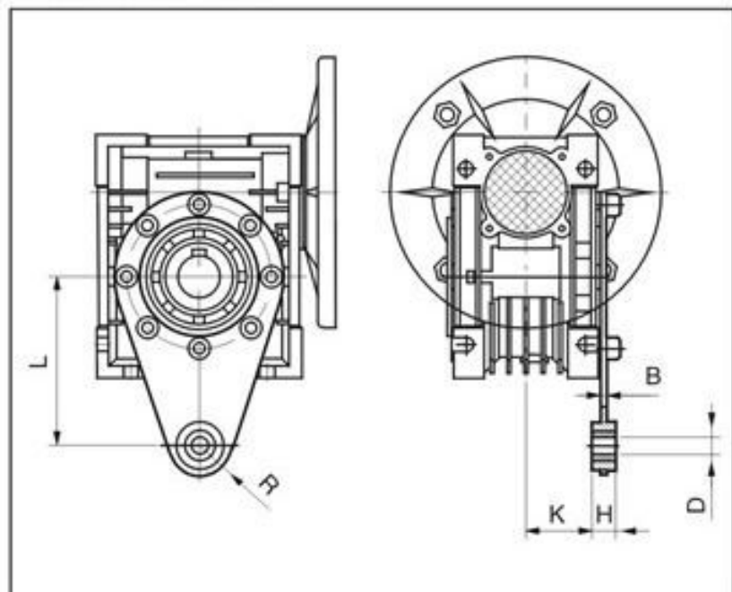
扭力臂 (A) 尺寸
