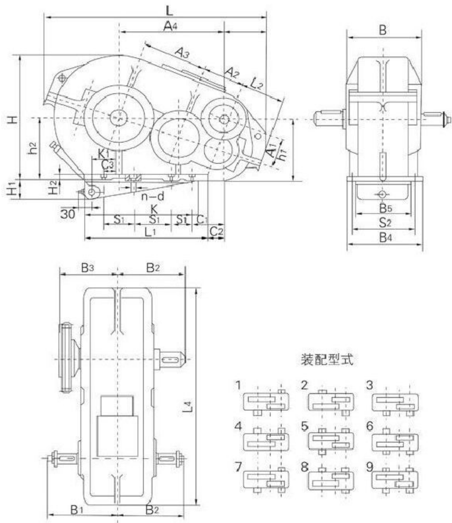
ZQ型卧式渐开线圆柱齿轮大传动比减速机外形及安装尺寸
